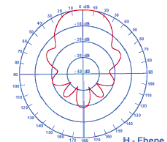
H - Ebene
